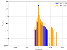
(n) L2-ER: task 5
