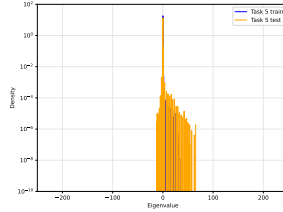
(e) BP: task 5
